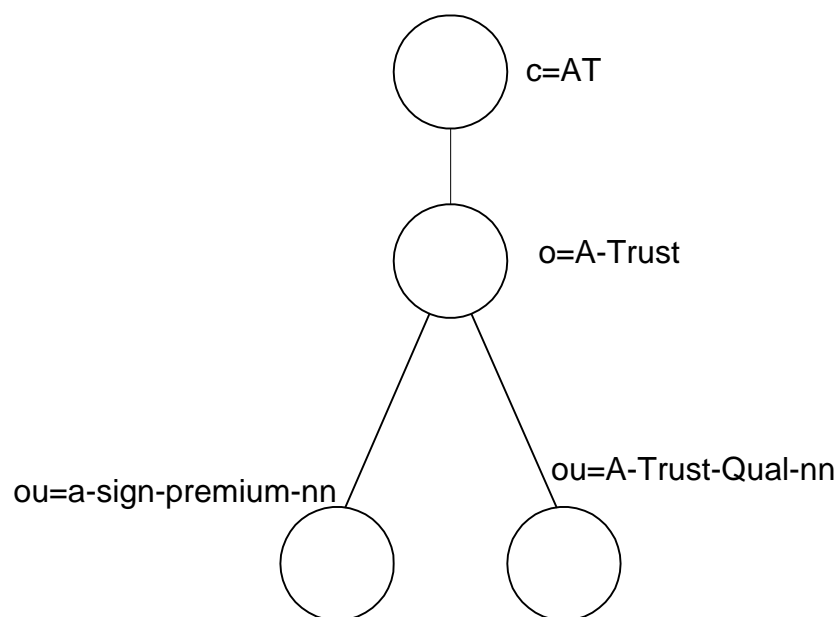
Abbildung 2 Verzeichnisbaum
