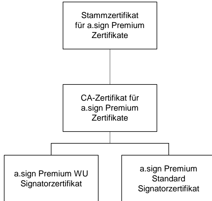
Abbildung 1 Zertifizierungshierarchie
