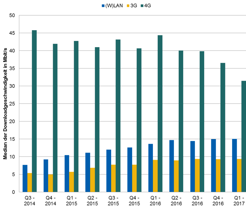
Abbildung 8: Median der Downloadgeschwindigkeit
