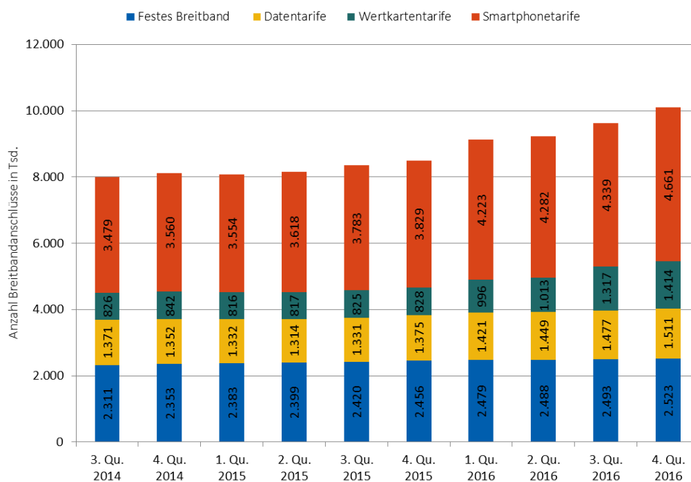
Abbildung 4: Breitbandanschlüsse im Fest- und Mobilnetz 8
