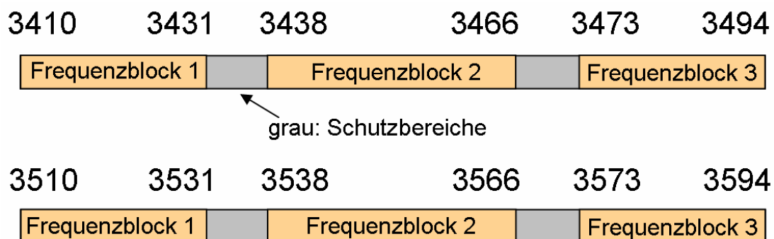
ABBILDUNG: ÜBERSICHT FREQUENZBLÖCKE 1-3 UND SCHUTZBEREICHE 1-2 UND 2-3
